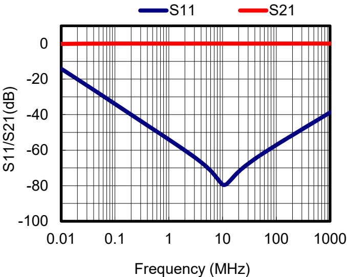
S parameters(Series)
