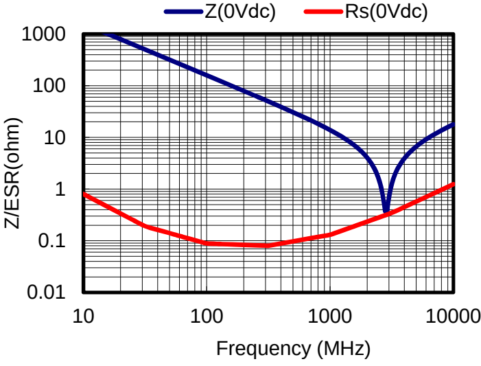
Impedance/ESR
