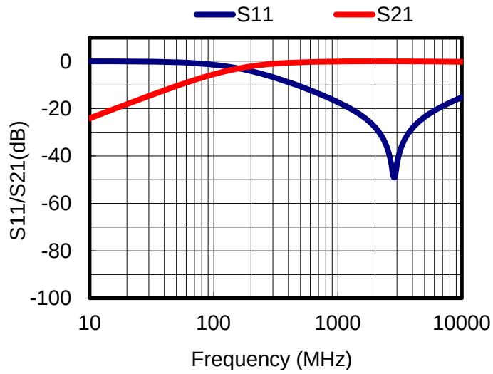
S parameters(Series)
